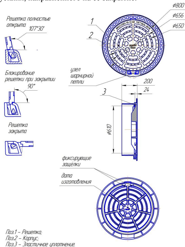
Рисунок 1. Дождеприемник ДМ2(С250)-10-12-60
