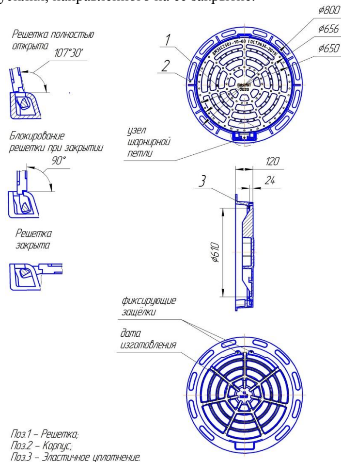
Рисунок 1. Дождеприемник ДМ2(С250)-10-60
