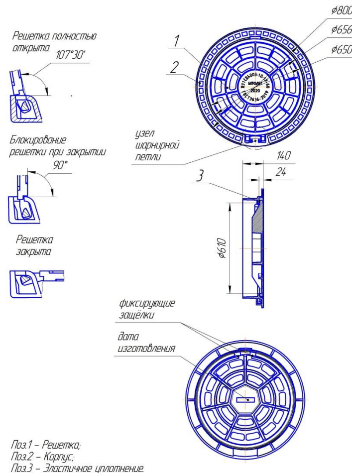
Рисунок 1. Дождеприемник ДУ1(Д400)-10-12-60
