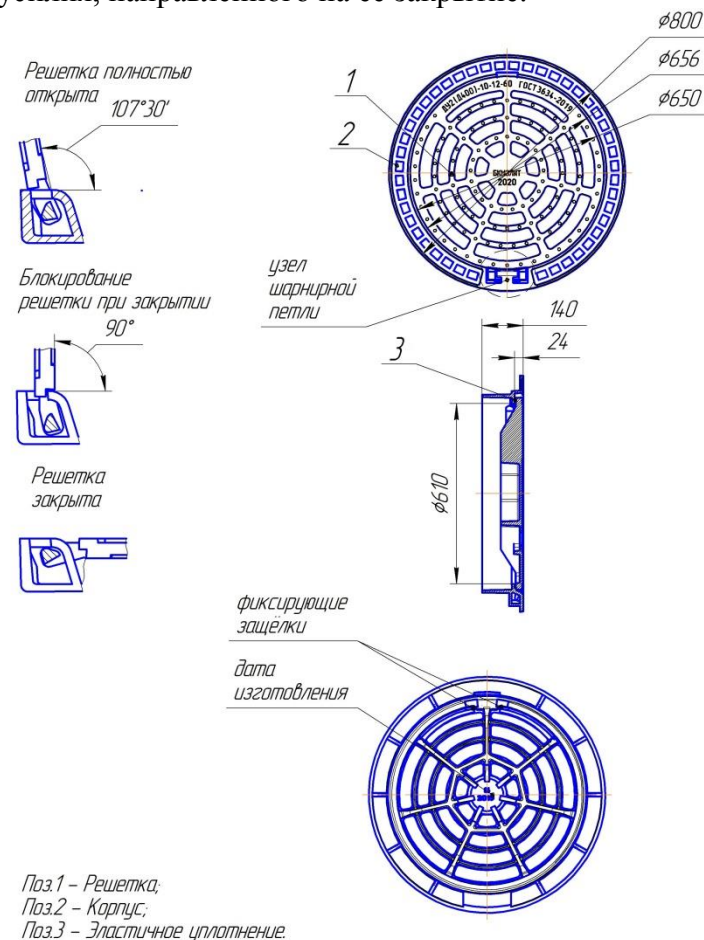
Рисунок 1. Дождеприемник усиленный ДУ2(Д400)-10-12-60 (140)
