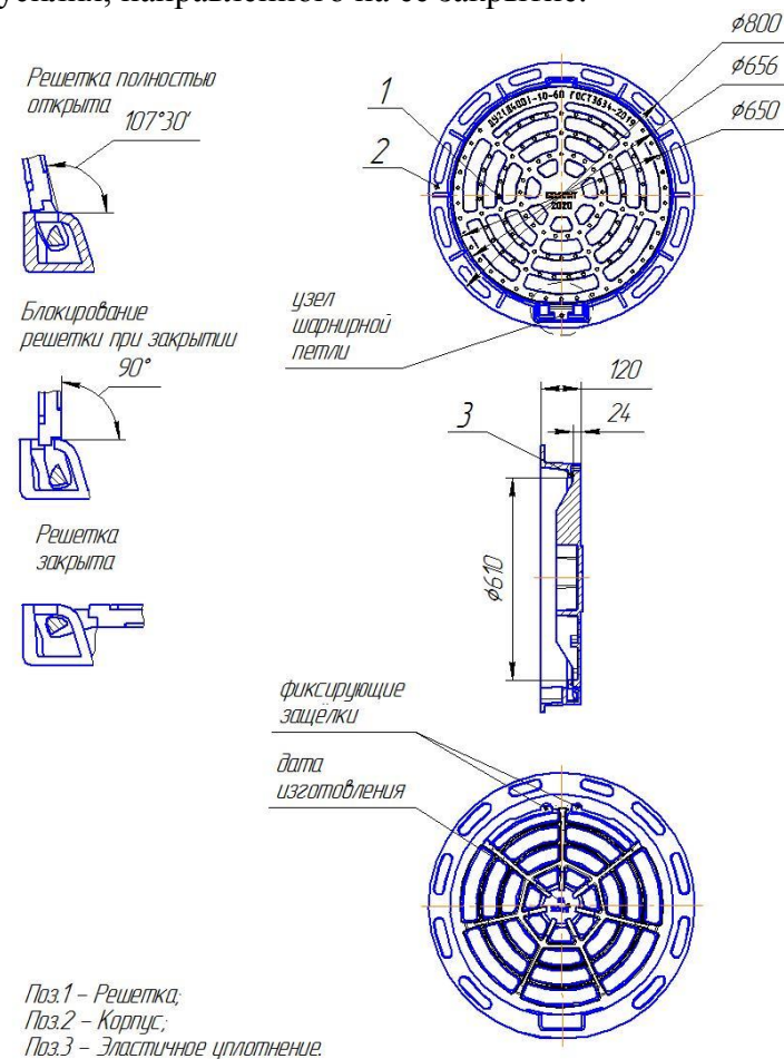
Рисунок 1. Дождеприемник усиленный ДУ2(Д400)-10-60 (120)
