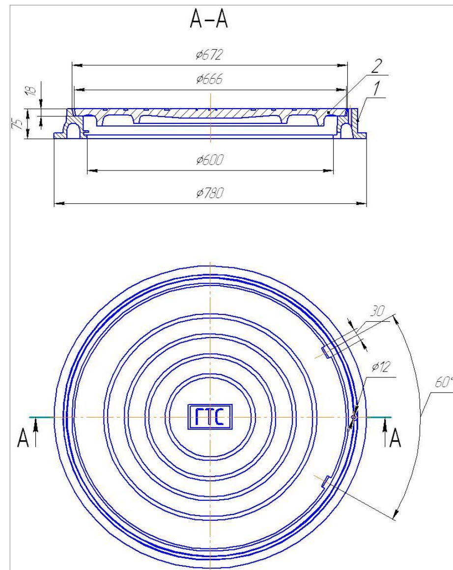
Рис.1. Люк канализационный общего назначения ГТС-Л
