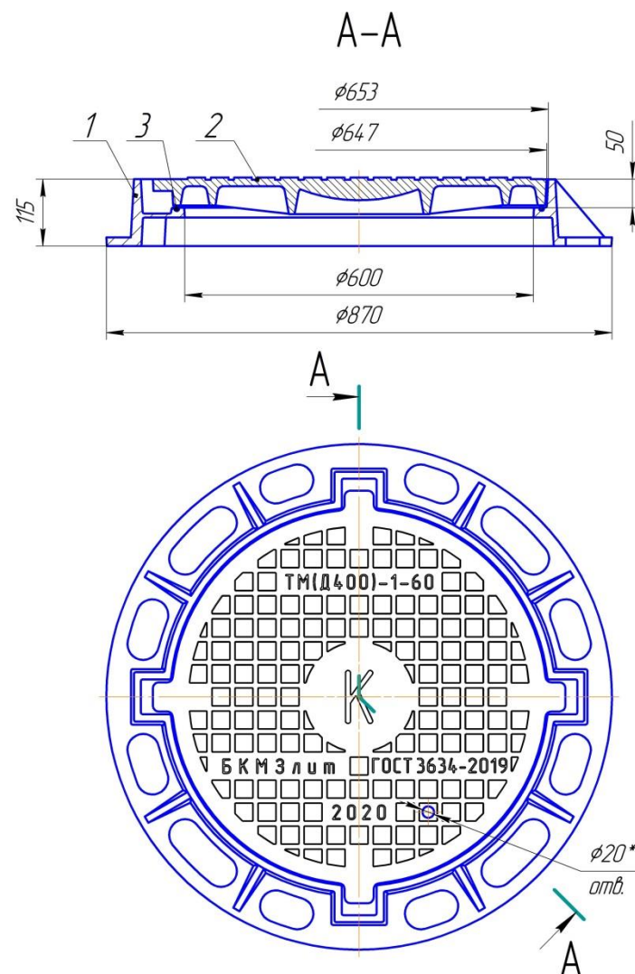
Рис.1. Люк тяжелый магистральный ТМ-Д400-1-60
