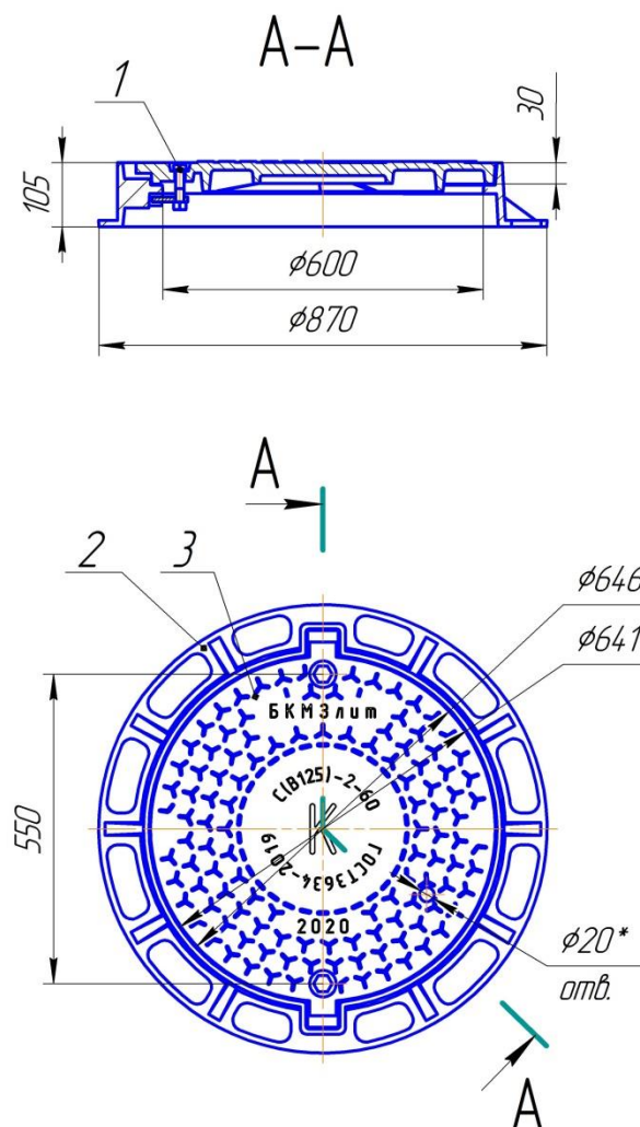
Рис.1. Люк средний С(В125)-2-60 (с запорным устройством)
