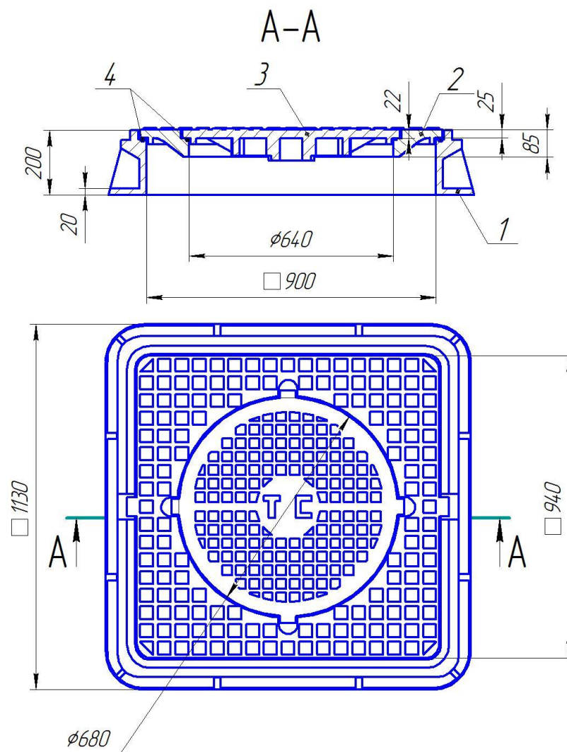
Рис.1. Люк канализационный общего назначения ТС-0298-250
